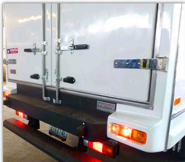
Bisagras de acero de 3"x 3/8", para máxima resistencia.
